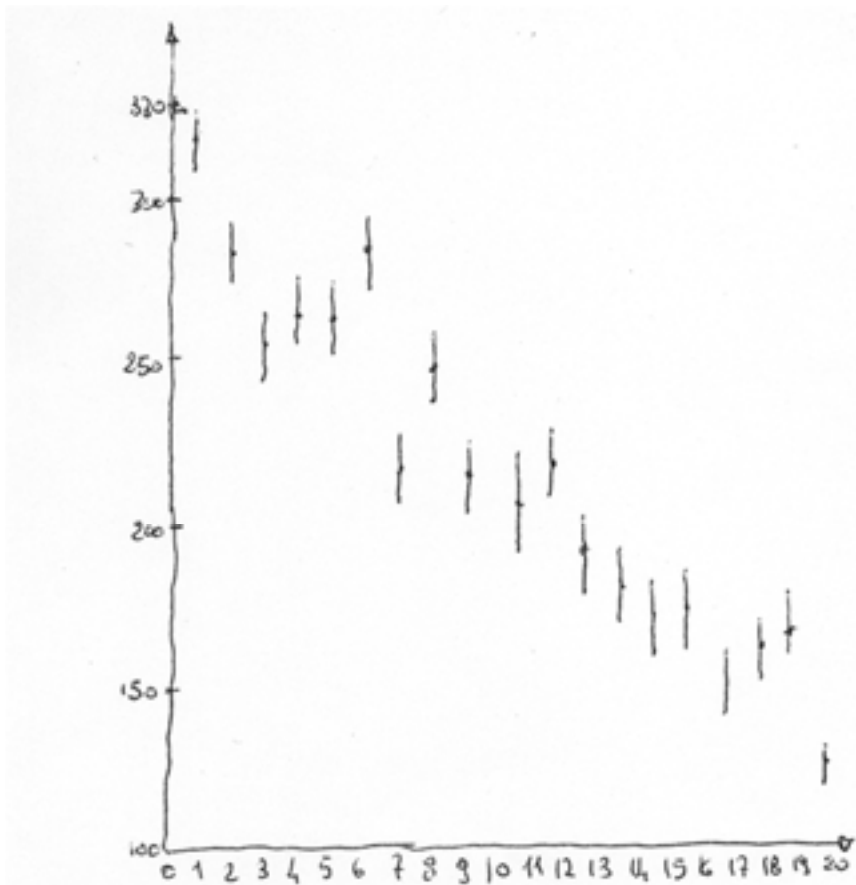
Fig 3 Sb (ossido) decadimento dopo l'attivazione (beta)
