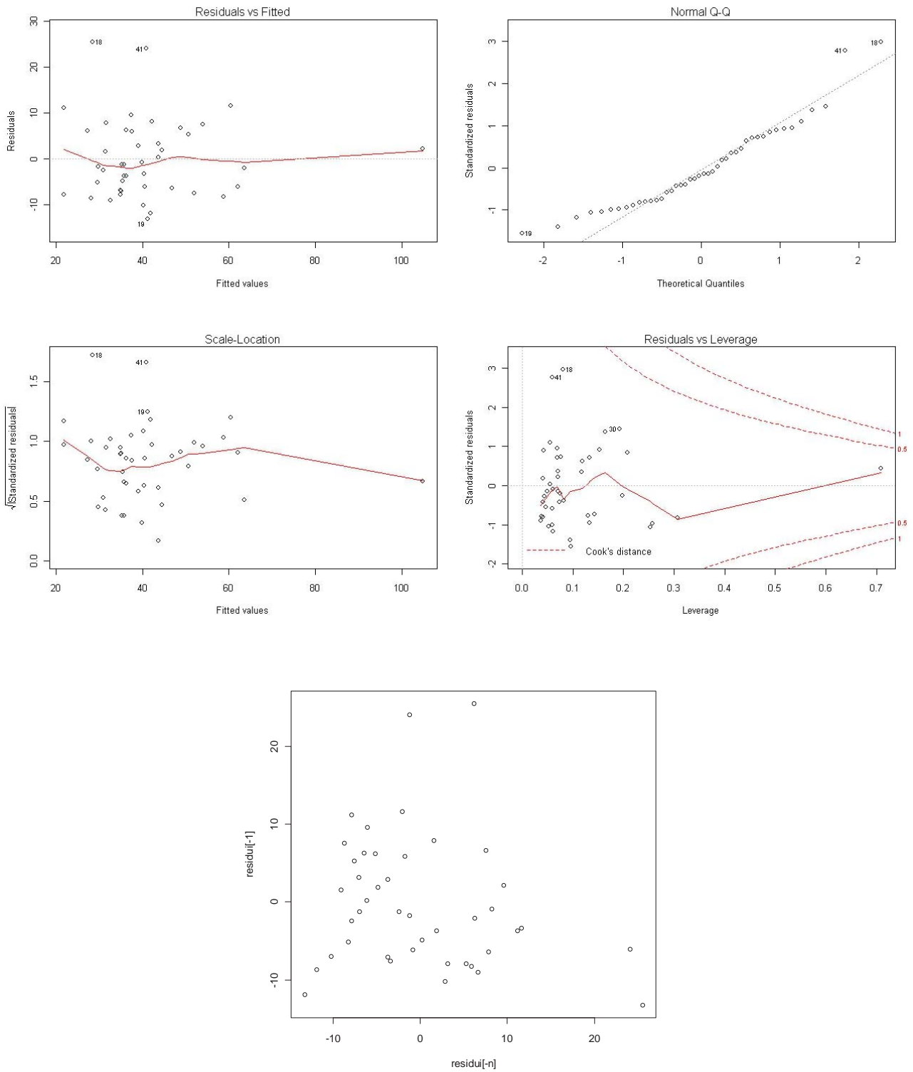
Fig.3 Verifica grafica degli assunti di base del modello di regressione [3]
