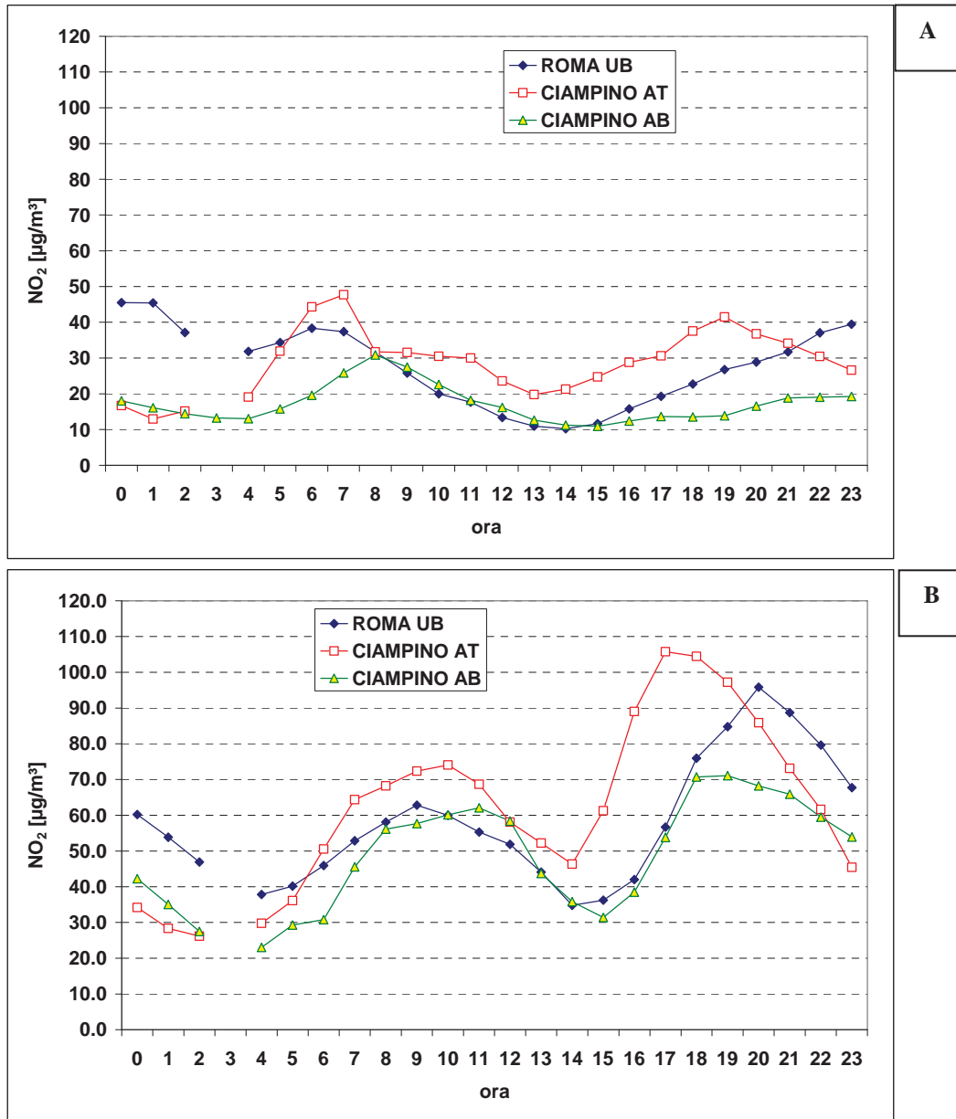
Figura 2. “giorno tipo” dell’NO 2 differenziato per stagione (A=estiva, B=invernale) e per sito (Ciampino, AT vs Roma UB)
