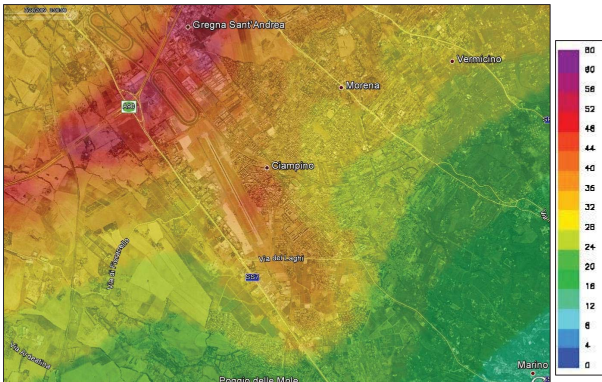
Figura 5. Mappa di concentrazione media di NO 2 (µg/m 3 ) prodotta dal Sistema NRT (01-15 giugno 2011).
