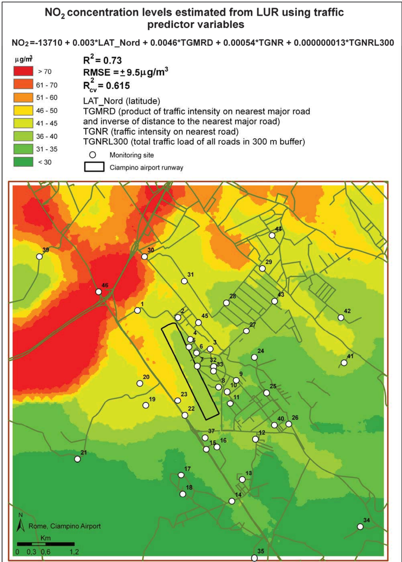
Fig.4 Variabilità spaziale dei livelli di concentrazione di NO 2 nell'intorno dell'aeroporto di Ciampino
